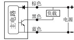
NPN型
